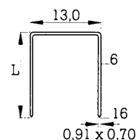
Agrafe du type 380
