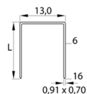
Agrafe du type 80 et 380
