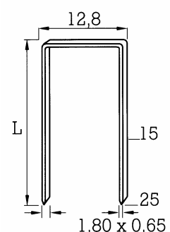
Agrafe type 195
