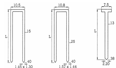
Agrafes du type 14 et 155 et clou en T
