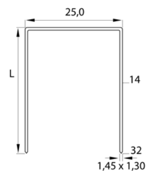
Agrafe type 140
