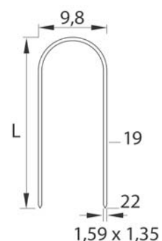
Agrafe type 150
