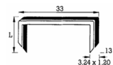
Agrafe EPAL type 33
