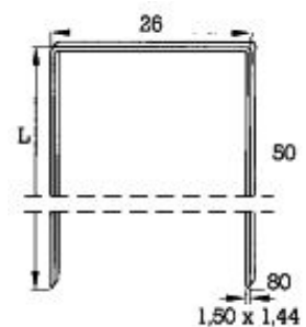
Agrafe type 146
